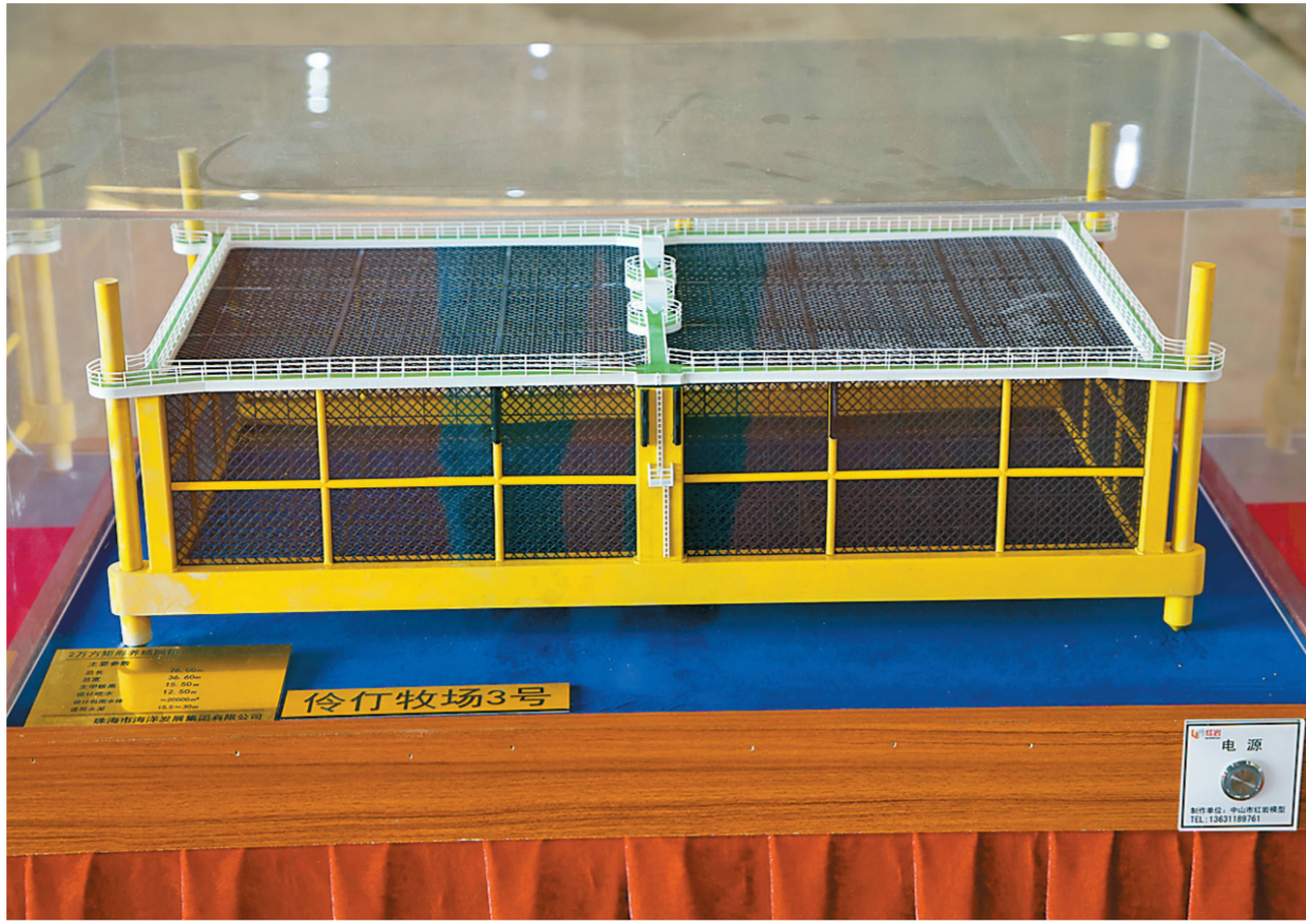
伶仃牧场3号矩形养殖网箱模型。 本报记者 李建束 摄
